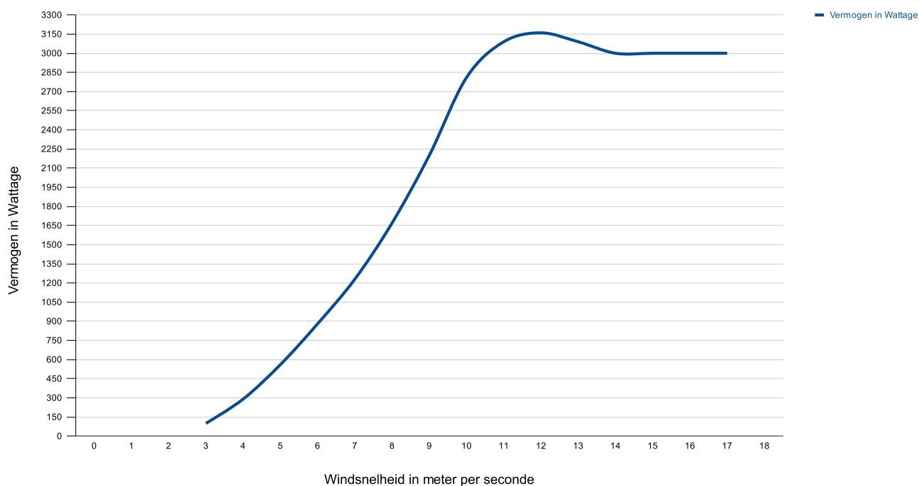
3 kW windmolen geschatte opbrengst per M/S per uur
