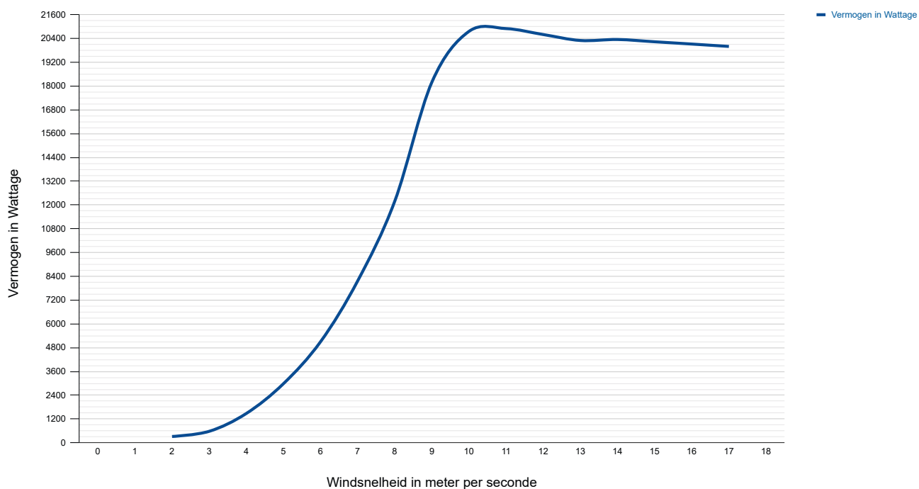
20 KW active pitch windmolen geschatte opbrengst per M/S per uur
