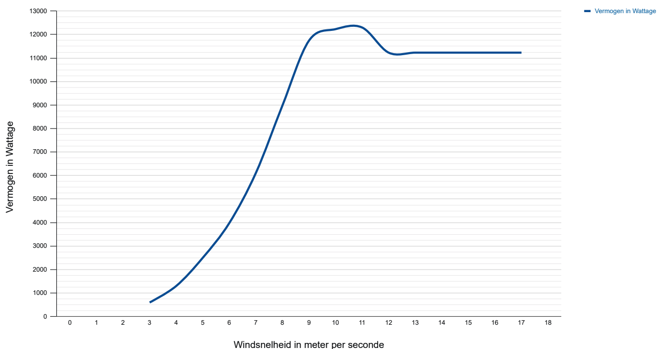
10 KW active pitch windmolen geschatte opbrengst per M/S per uur
